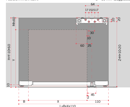
POSIÇÃO DE ABERTURA TOTAL / TOTAL OPENING POSITION / POSICION TOTAL DE APERTURA
