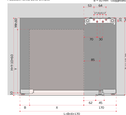
POSIÇÃO DE ABERTURA TOTAL / TOTAL OPENING POSITION / POSICION TOTAL DE APERTURA
